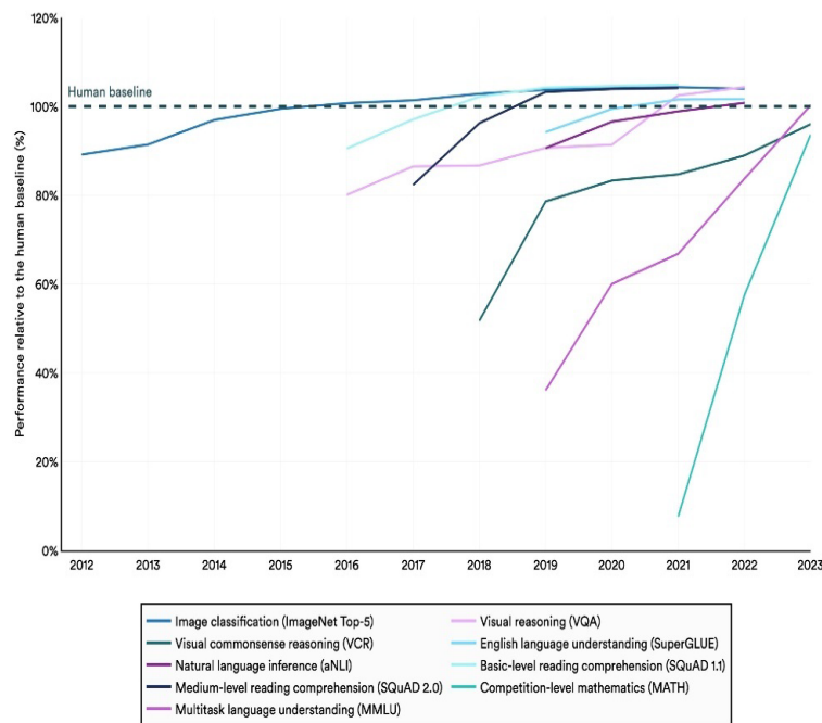
Figura 1. Rendimiento técnico de la IA. Medidas seleccionadas, 100%= referencia humana
